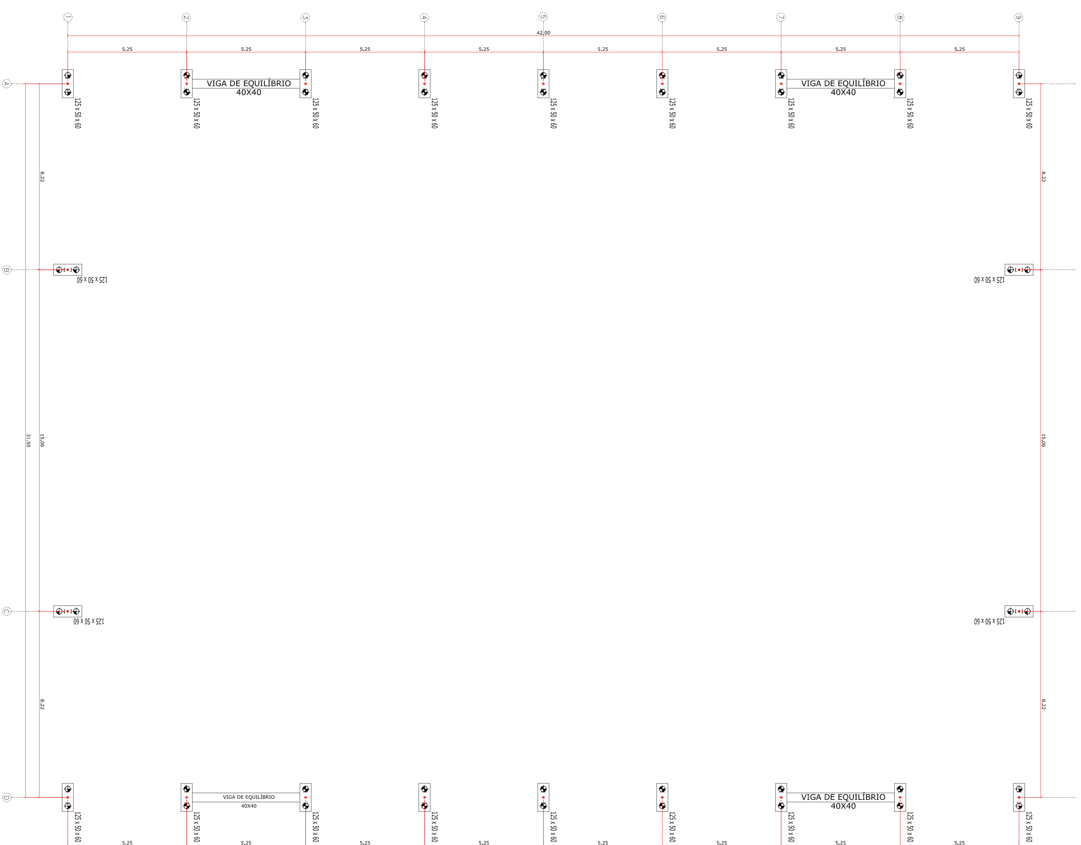
PLANTA DE FORMA – FUNDAÇÃO ESCALA 1:100
